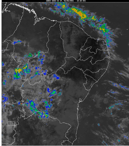
Imagem do satélite GOES – dia 04/02/2021 às 09h40min Fonte:
