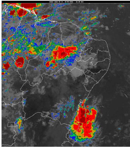
Imagem do satélite GOES – dia 15/03/2022 às 09h20min Fonte:
