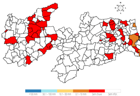
PRECIPITAÇÃO MÁXIMA DOS MUNICÍPIOS/POSTOS NO DIA 05/06/2023
